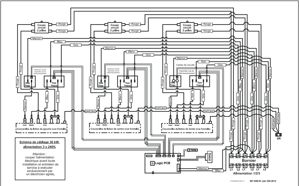
Fig. 3 Schéma de câblage interne pour l'unité monophasée WH36 unit.
