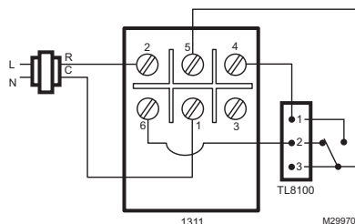
Fig. 20. Schéma de câblage pour la vanne 1311 White Rogers.
