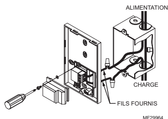
Fig. 13. Acheminement des fils vers le thermostat.
