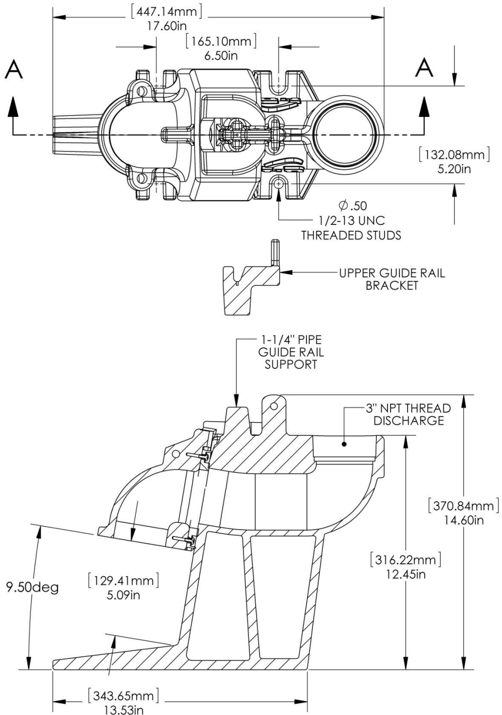
SECTION A-A SCALE 1 : 4.3
