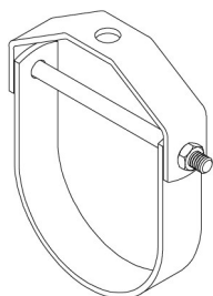
FIG. 420 A.W.W.A. CLEVIS PAGE 47
