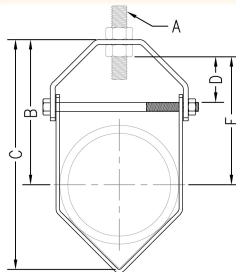
FIG. 450V
