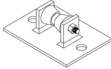
FIG. 486 PIPE ROLLER STAND PAGE 60
