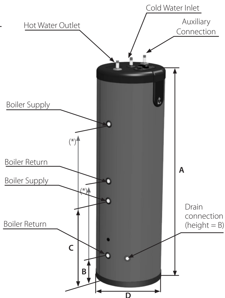
Fig. 25 - GINIUS 65 Dimensions
