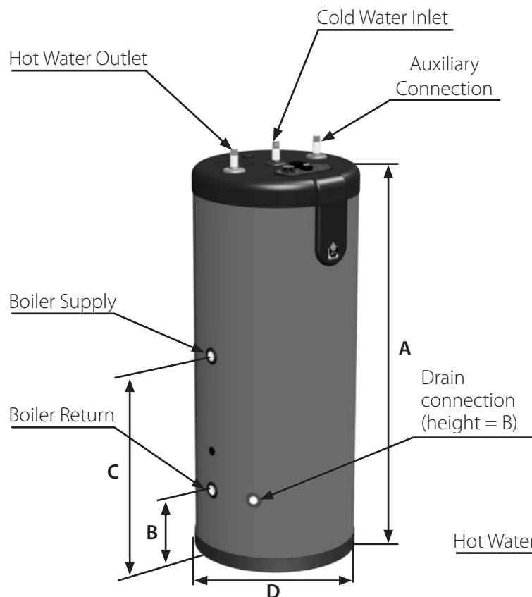
Fig. 24 - GINIUS 35-45-55 Dimensions
